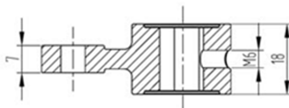
截面 A-A
